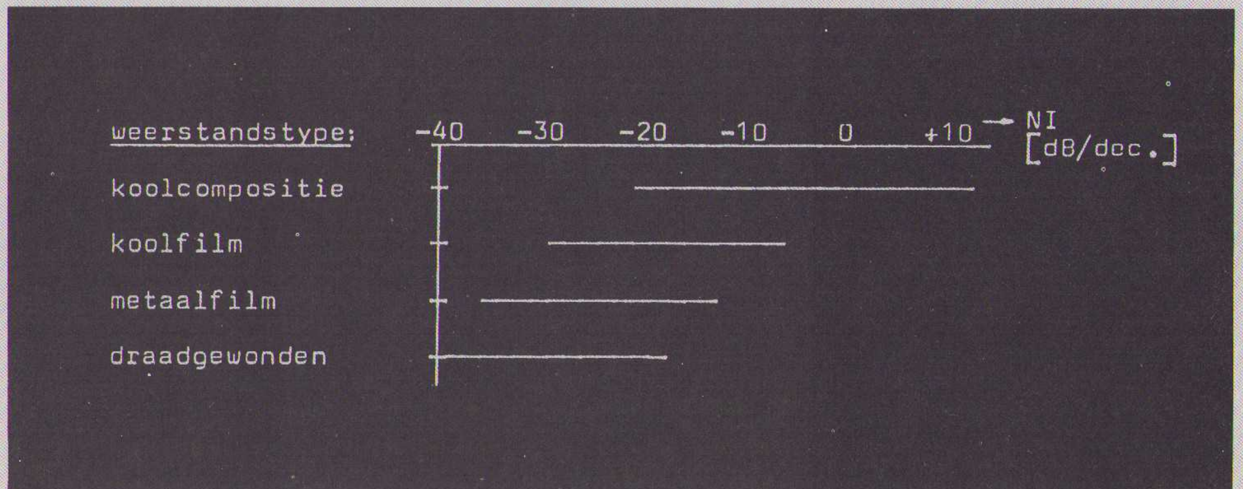
Figuur 1.3.2.3. Overzicht van ruisindices van verschillende typen weerstanden.
